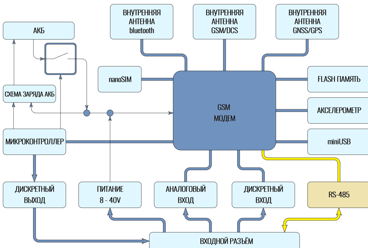
Рисунок 1.3 Блок-схема навигационного терминала УМКа312
