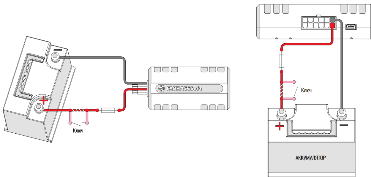
Рисунок 2.8 Подключение питаниям (310 – слева; 312 -справа)
