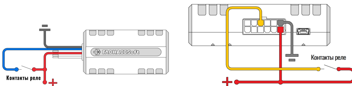
Рисунок 2.13 Варианты подключения дискретных датчиков
