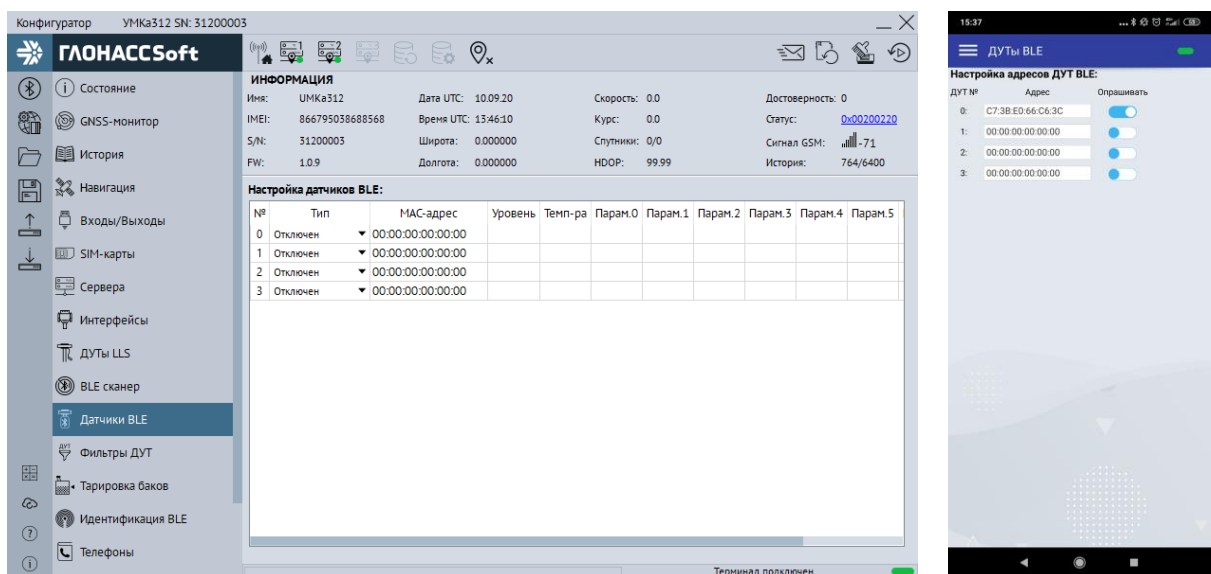
Рисунок 3.25 Вкладка «Дуты BLE»
