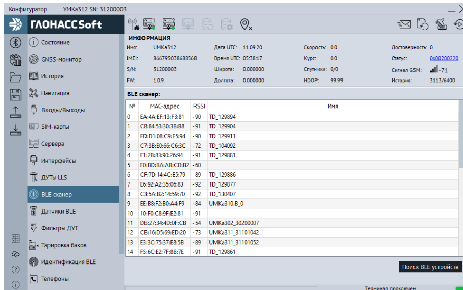
Рисунок 3.24 Вкладка «BLE сканер»
