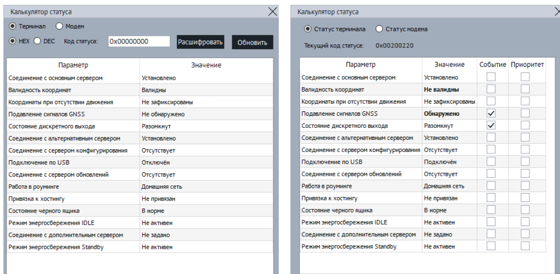
Рисунок 3.15 Калькулятор статуса
