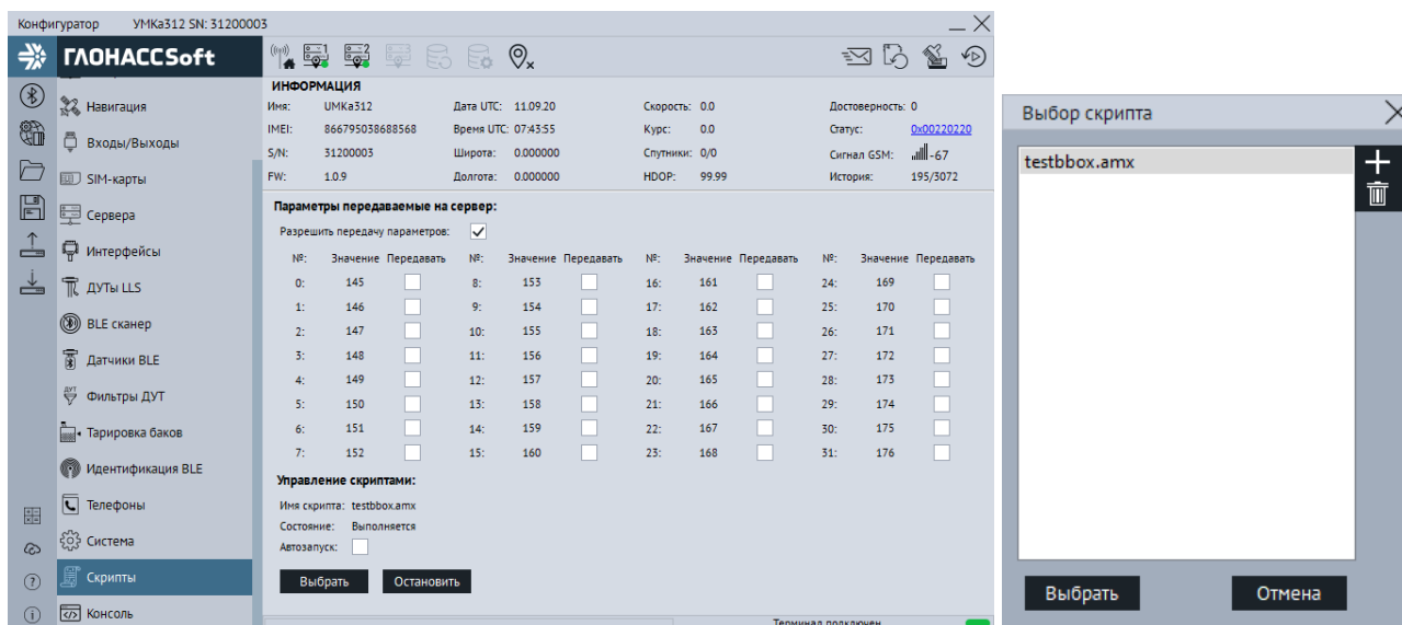
Рисунок 3.31 Вкладка «Скрипты»
