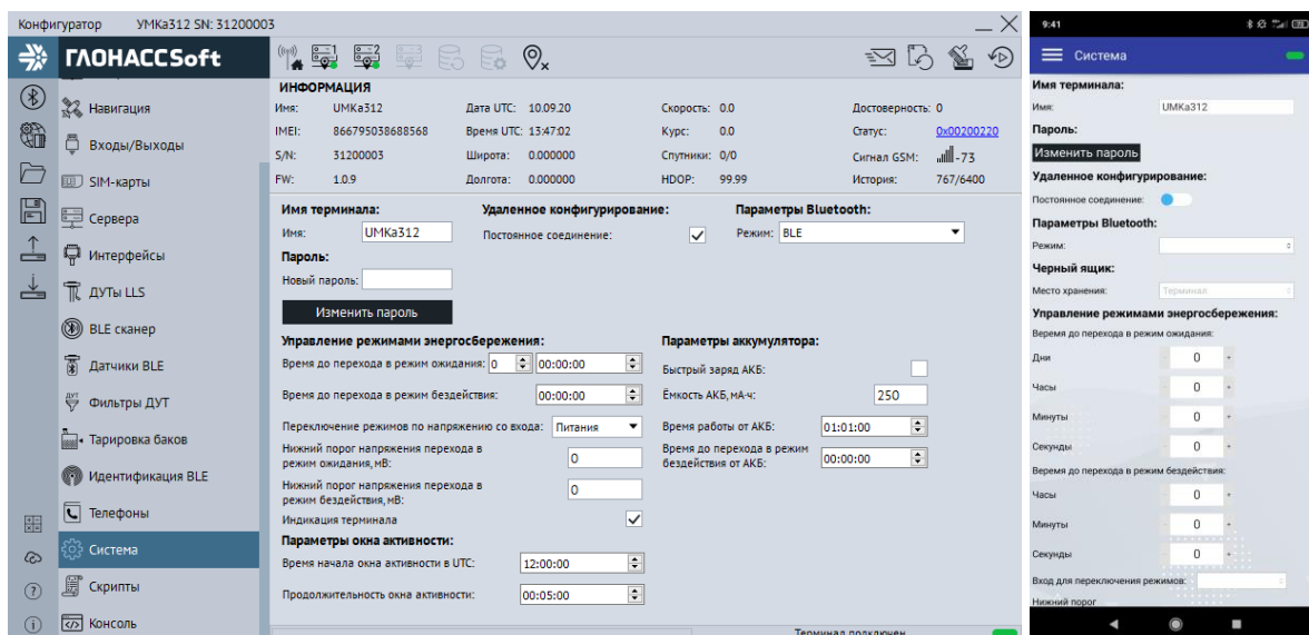
Рисунок 3.30 Вкладка «Система»
