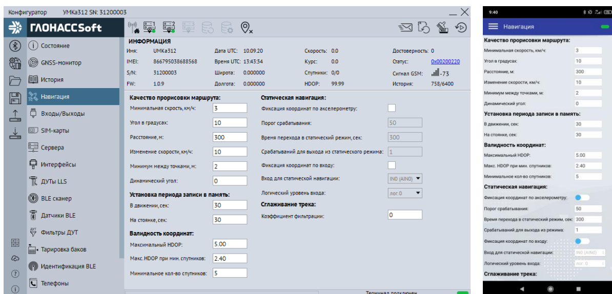
Рисунок 3.17 Вкладка «Навигация»
