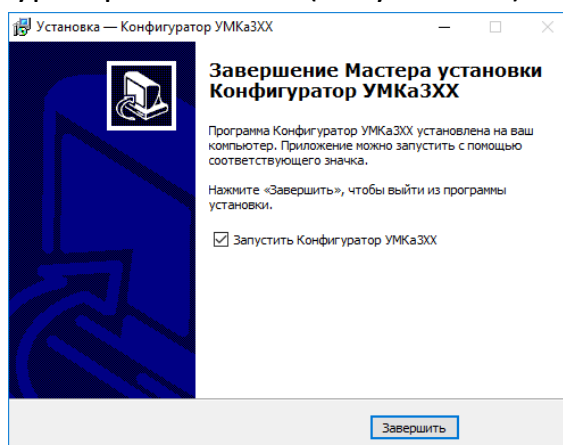
Рисунок 3.8 Запуск приложения
