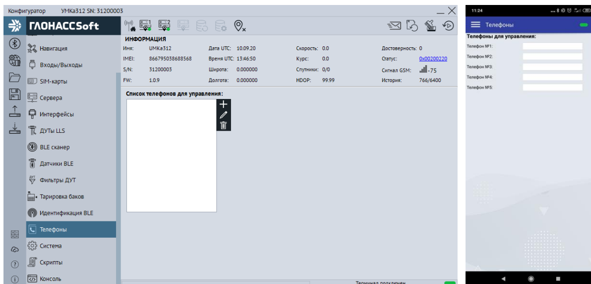
Рисунок 3.27 Вкладка «Телефоны»
