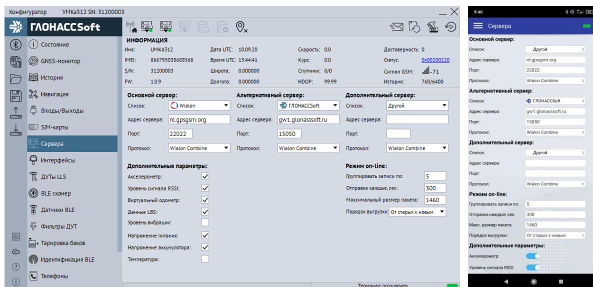
Рисунок 3.21 Вкладка «Сервера»
