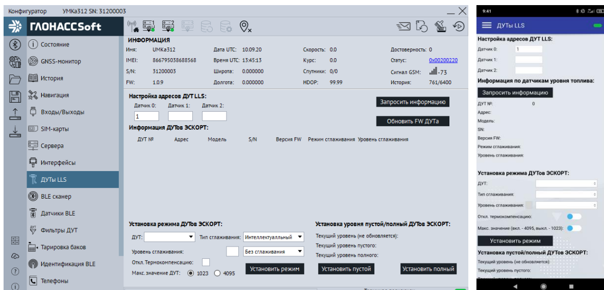
Рисунок 3.23 Вкладка «ДУТЫ»
