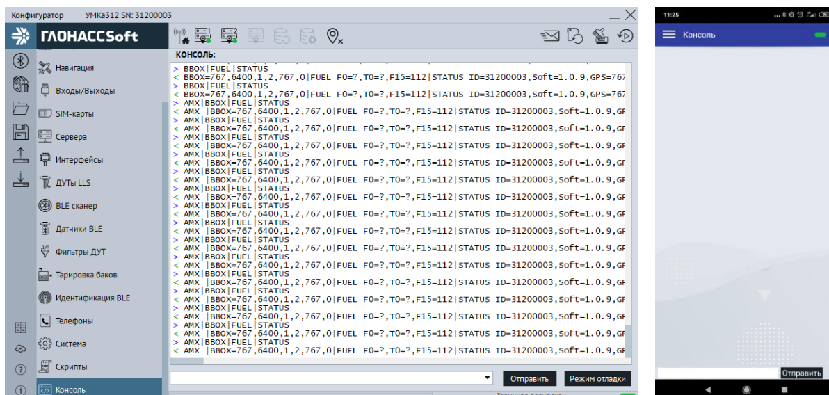
Рисунок 3.32 Вкладка «Консоль»
