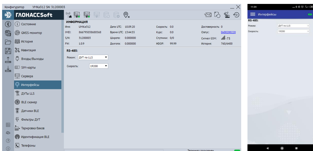
Рисунок 3.22 Вкладка «Интерфейсы»
