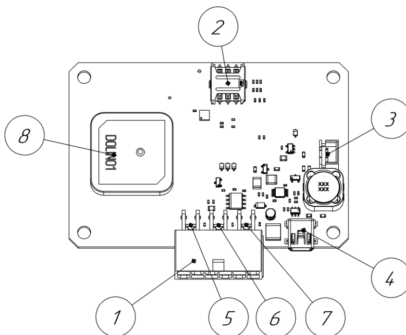
Рисунок 2.2 Основные элементы терминала
