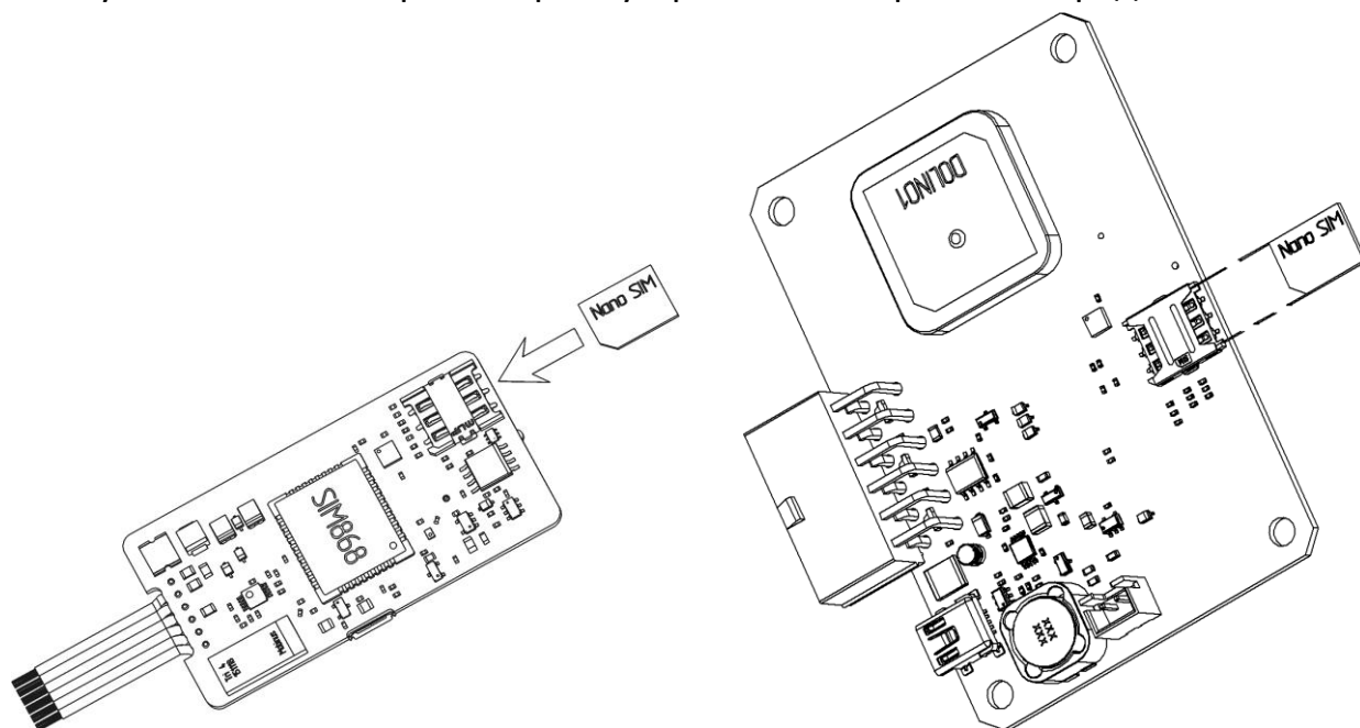
Рисунок 2.6 Установка SIM-карты (310 – слева; 312 - справа)
