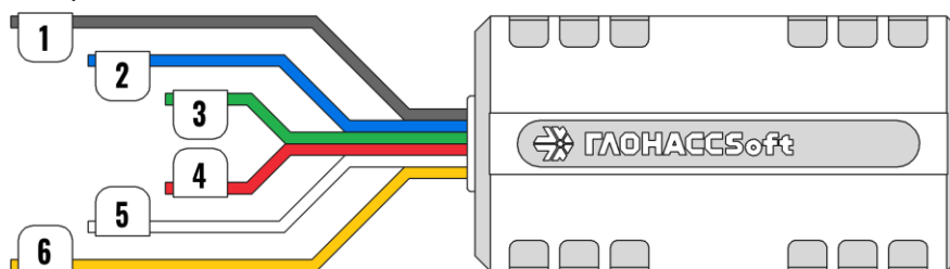
Рисунок 2.3 Нумерация выводов УМКа310
