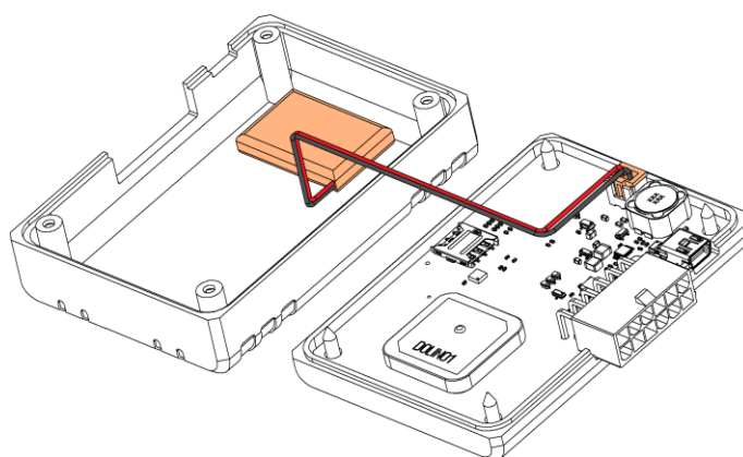
Рисунок 2.7 Установка аккумулятора
