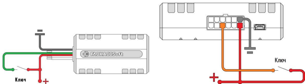
Рисунок 2.11 Подключение с подтяжкой к «-» (310 – слева; 312 - справа)
