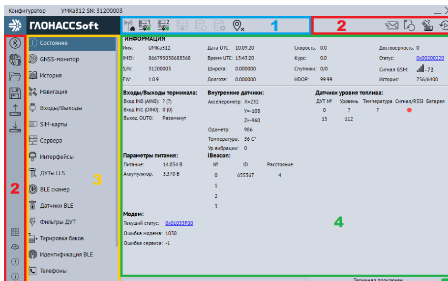
Рисунок 3.9 Стартовое окно «Состояние»
