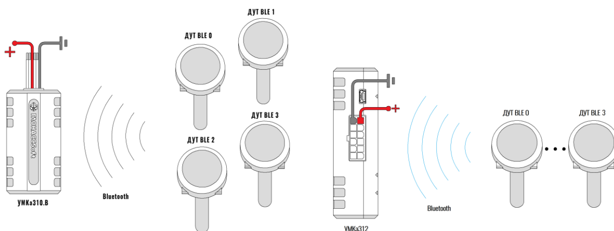
Рисунок 2.18 Подключение ДУТ по BLE (310 – слева; 312 - справа)
