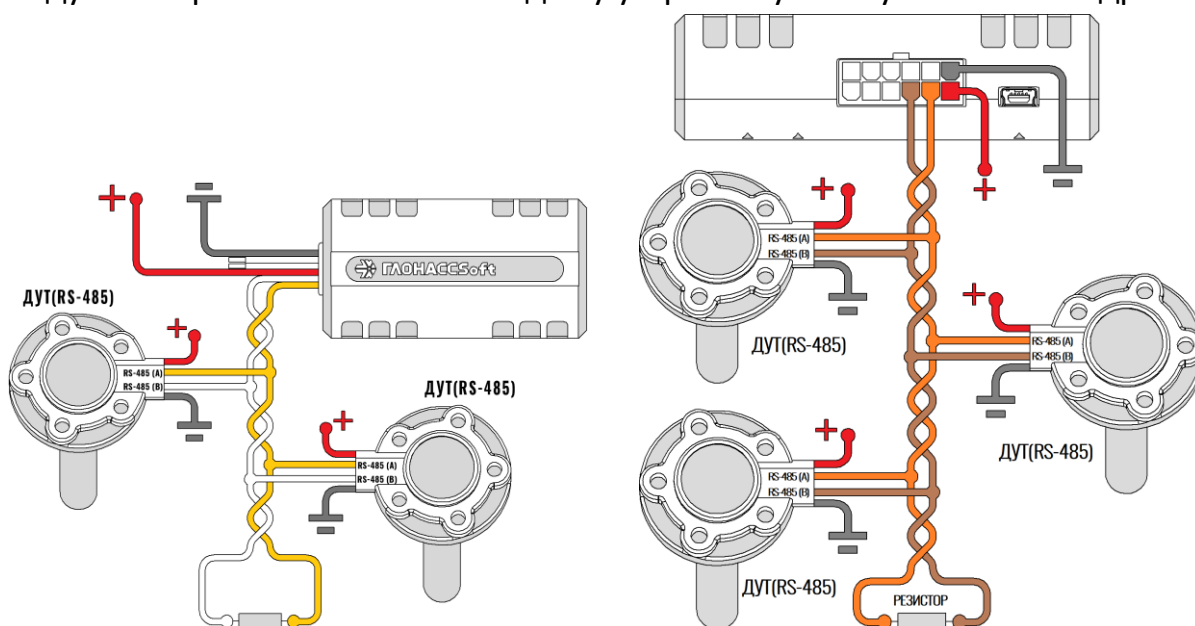
Рисунок 2.16 Подключение ДУТ по интерфейсу RS-485 (310 – слева; 312 - справа)
