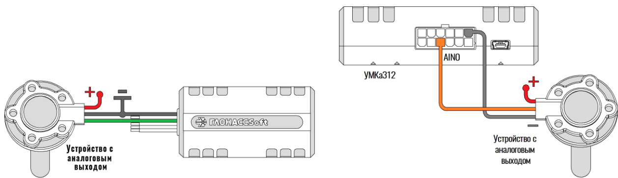
Рисунок 2.9 Подключение аналоговых источников (310 – слева; 312 - справа)
