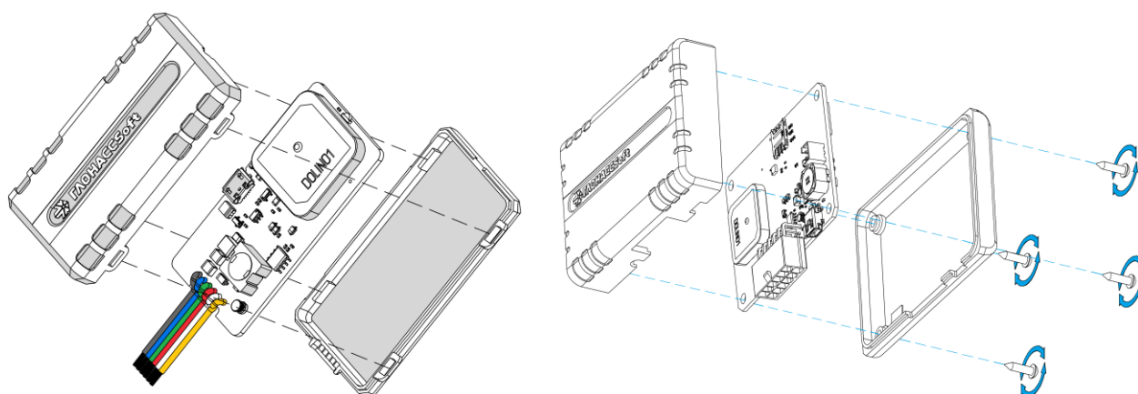
Рисунок 2.5 Вскрытие корпуса терминала (310 – слева; 312 - справа)
