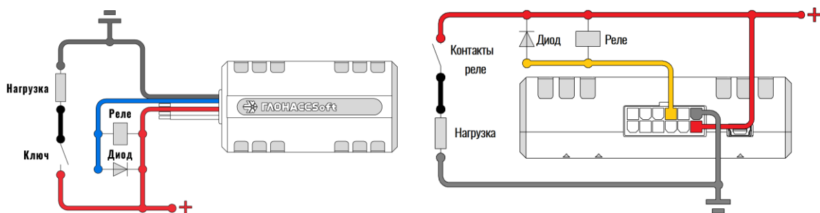
Рисунок 2.15 Подключение мощной нагрузки (310 – слева; 312 - справа)
