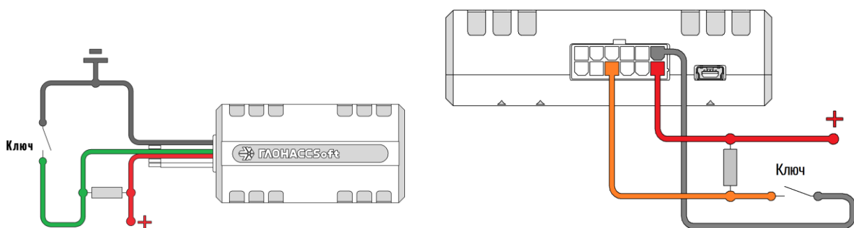
Рисунок 2.10 Подключение с подтяжкой к «+» (310 – слева; 312 - справа)
