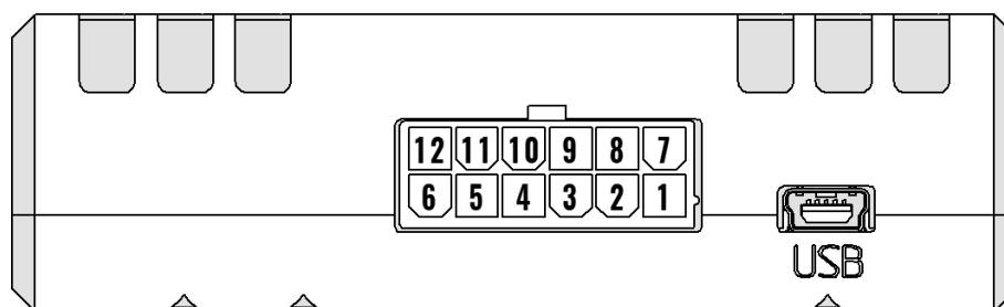
Рисунок 2.4 Нумерация выводов УМКа312
