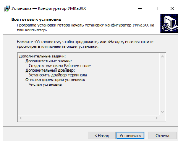
Рисунок 3.7 Начало установки
