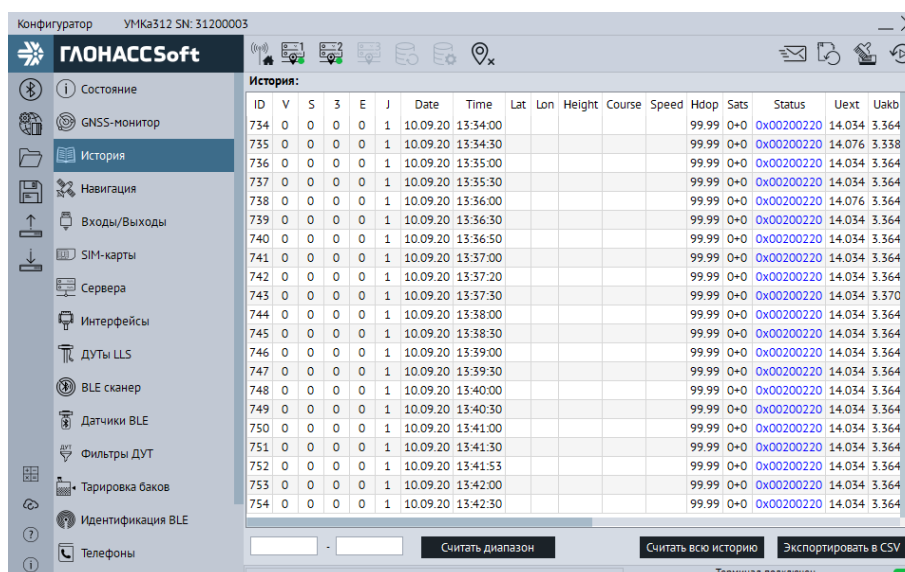
Рисунок 3.16 Вкладка «История»
