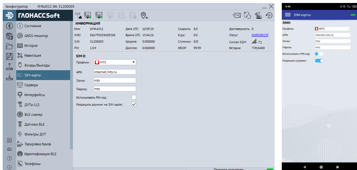
Рисунок 3.20 Вкладка «SIM-карты»
