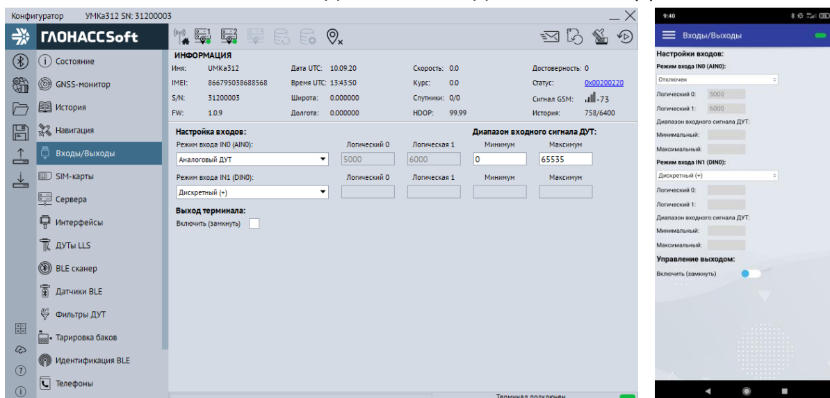
Рисунок 3.19 Вкладка «Входы/Выходы»
